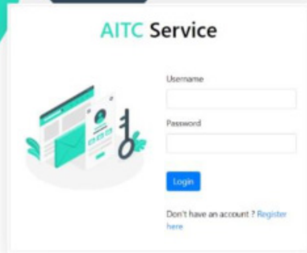
LOGIN
